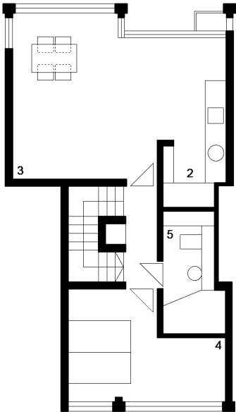
PLANTA SUPERIOR
